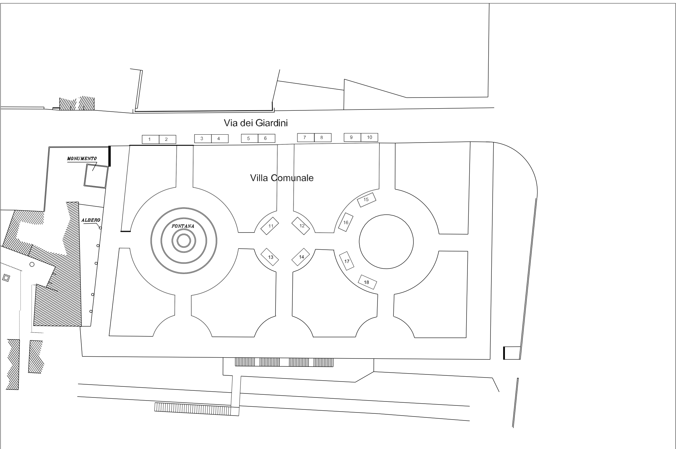
PLANIMETRIA DISLOCAZIONE N° 20 STANDS IN LEGNO DIM. 2X4 mt
